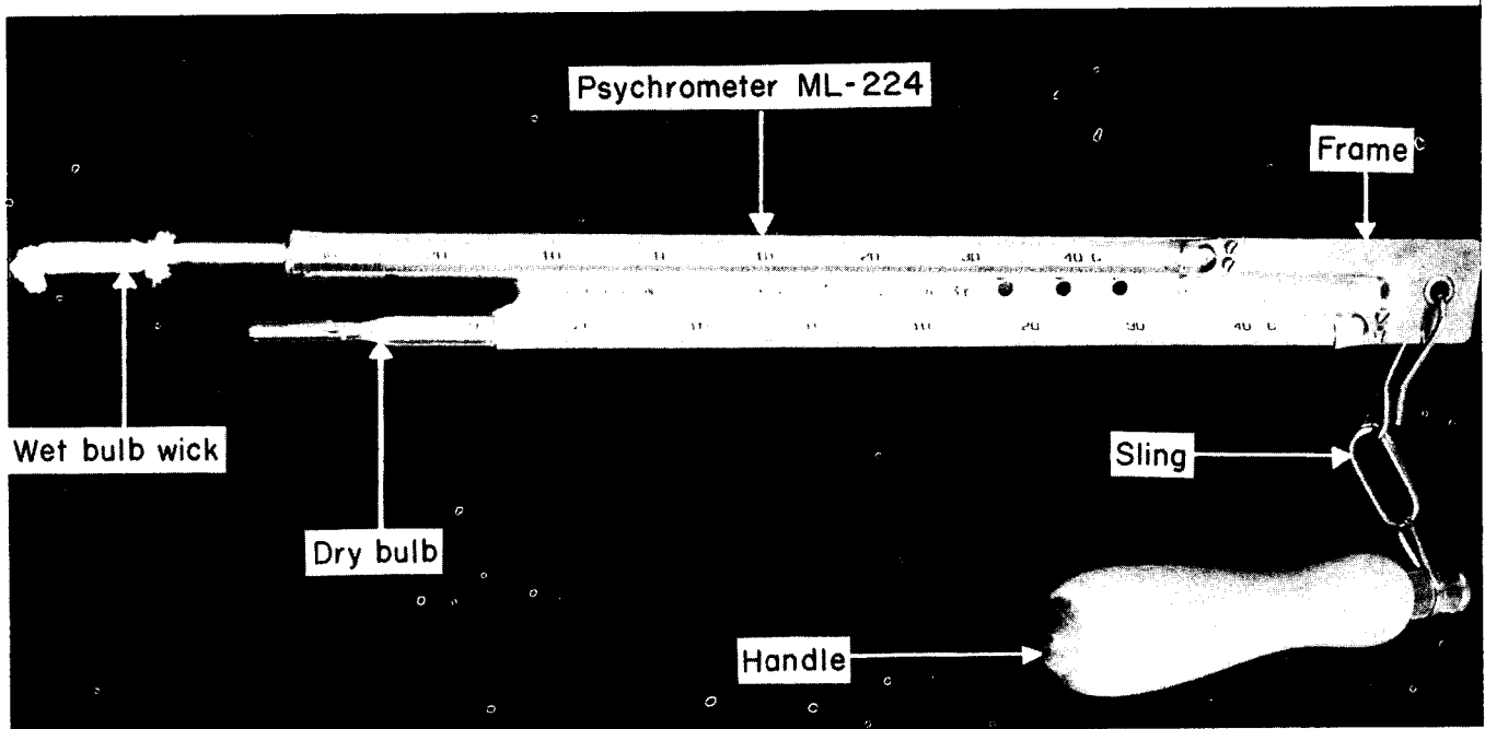
Figure 28. Psychrometer ML-224.
